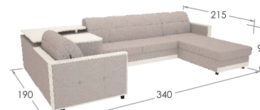
7.12 П-ОБРАЗНЫЙ ДИВАН / FLAT-TOPPED SOFA СП. МЕСТО / SLEEPING PLACE 205x225
