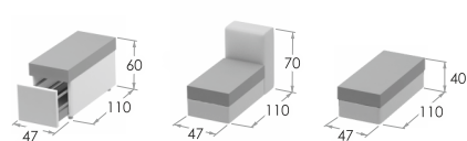
БАР С ВЫКЛЮЧНЫМ ЯЩИКОМ / BUILT-IN BAR
