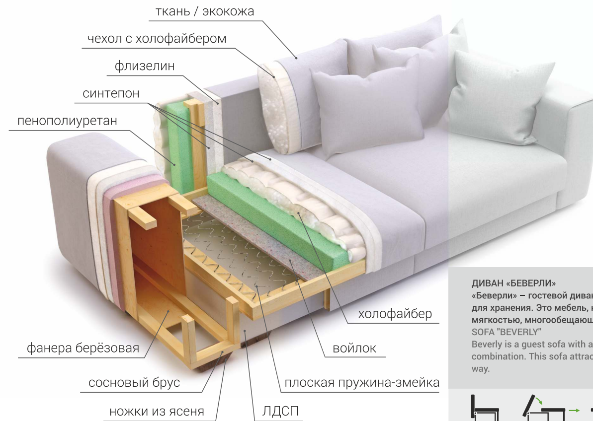
20.1 ■ ПРЯМОЙ ДИВАН / FLAT SOFA СП. МЕСТО / SLEEPING PLACE 203x170
