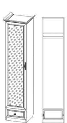
Р 330.09 Шкаф с витриной 2172x534x466
