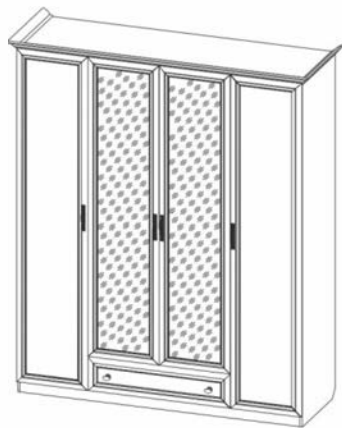
Р 330.32 Шкаф для одежды 2172x534x608
