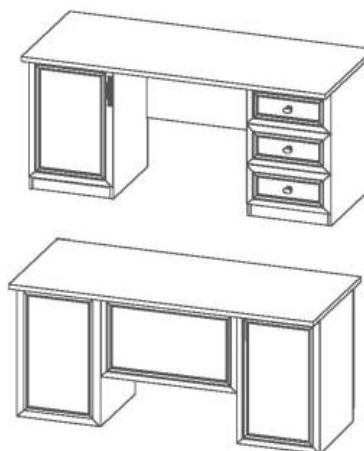
выс./шир./глуб. 738x1600x700
