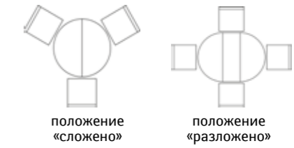
Стол «Валенсия 11» П358.07: L1000/1350xВ1000xН778
