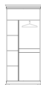
Шкаф «Верди Люкс 2/2» П487.35: L1148xВ477xН1996 (с выдвигной штангой для плечиков)
