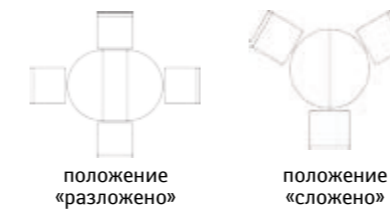
Стол «Верди 12А» П318.07: L1100/1450xВ1100xH778
