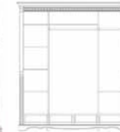
Шкаф для одежды 4д «Паола 2164-01» БМ671: L1858 x В678 x H2107 Шкаф для одежды 4д «Паола 2581-01» БМ671: L1858xВ678xH2250
