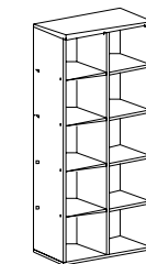
Шкаф П034.12C: L914xB443xH2105
