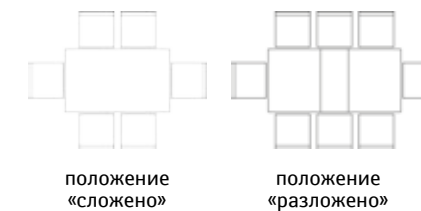
Стол раздвижной П607.05: L1600xB900xH777 в положении «разложено» L2100xB900xH777
