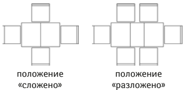
Стол «Поло 3Р» П257.08: L1500/1900xB900xH766
