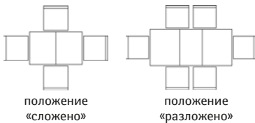
Стол «Поло 5» П257.07: L1300/1800xB800xH766
