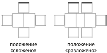
Стол «Альт 4» П285.06: L1080/1470xB670xH776
