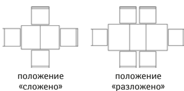
Стол «Альт 5» П285.07: L1330/1720xB720xH776
