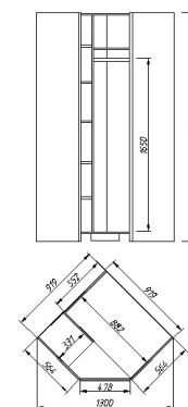
Шкаф для одежды ММ-346-01/04Б В1944 x Н2170 x Т581
