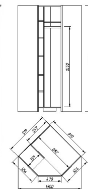
Шкаф для одежды ММ-341-01/08Б В981 x Н2229 x Т981
