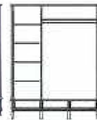
Шкаф ММ-267-01/03 В1771 x Н2238 x Т612
