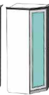
Шкаф для одежды ММ-341-01/08Б В981 x Н2229 x Т981
