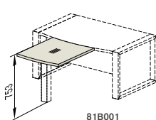
81B001 780x935x38
