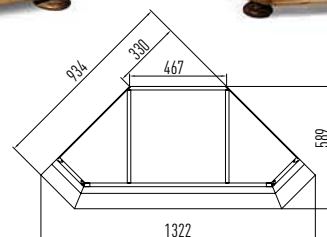
шкаф (угловой) ГМ 5613Е, 2114 x 1322 x 589
