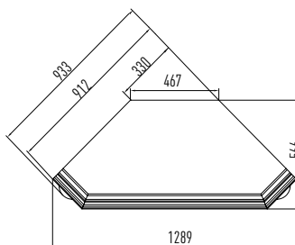
тумба (угловая) ГМ 5637, 843 x 1289 x 566
