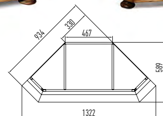
шкаф (угловой) ГМ 5613Е, 2114 x 1322 x 589
