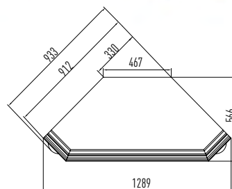
тумба (угловая) ГМ 5637, 843 x 1289 x 566
