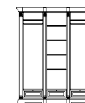
шкаф для платья и белья ГМ 5923, 2057 x 1614 x 673
