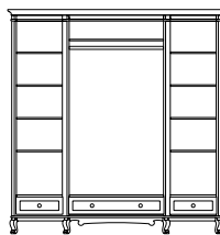
шкаф для платья и белья ГМ 5154, 2103 x 1995 x 622
